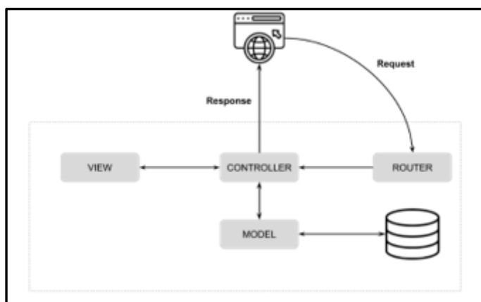
Рисунок 2 – Архитектура MVC
